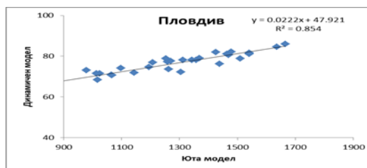
Фигура 1. Измерени стойности на чили единиците с Юта модел и Динамичен модел
