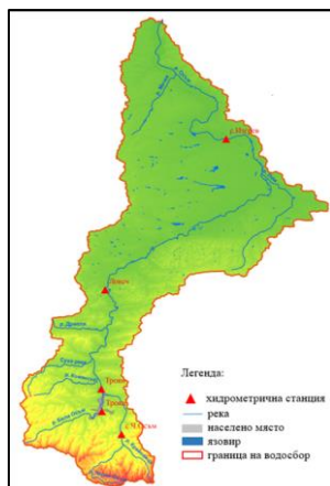
Фигура 2. Хидрометрични станции във водосбора на р. Осъм
