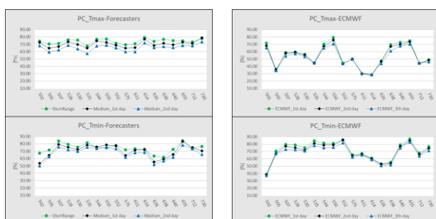
Фигура 1. PC на синоптиците и модела ECMWF за T_{\min} и T_{\max} в отделните точки
