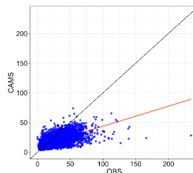
Фигура 2. Диаграма на разсейване на средноденоношните концентрации [ \mu\text{g m}^{-3} ] на ФПЧ 10
