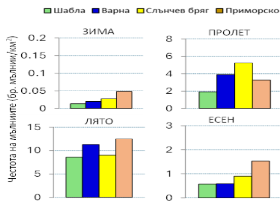
Фигура 1. Сезонна честота на мълниите (март 2005 – февруари 2015 г.) на „Шабла“, „Варна“, „Сл. бряг“ и „Приморско“
