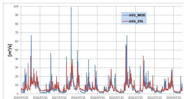
Фигура 2. Сравнение между осреднените измерени и моделирани редици ВК за 146 станции в България
