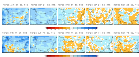
Фигура 5. Като фиг. 1, но по RCP2.6
