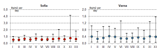
Фигура 1. Вариация във времето на средна, максимална и минимална 120-часова обща бета активност на отлагане върху планшет, 2024 г.
