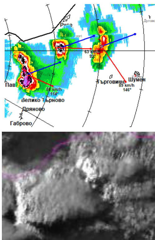
Фигура 1. Радарна и спътникова информация от 12.06.2024 в 18:30 LT (синя стрелка – вектор на водещ поток, червена стрелка – вектор на движение на бурята)
