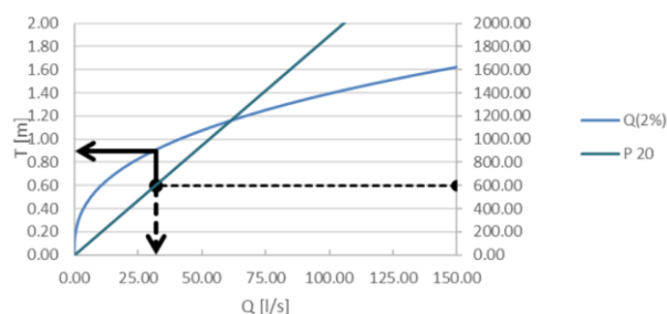
Фигура 3. Технология на изследването при задача 3
