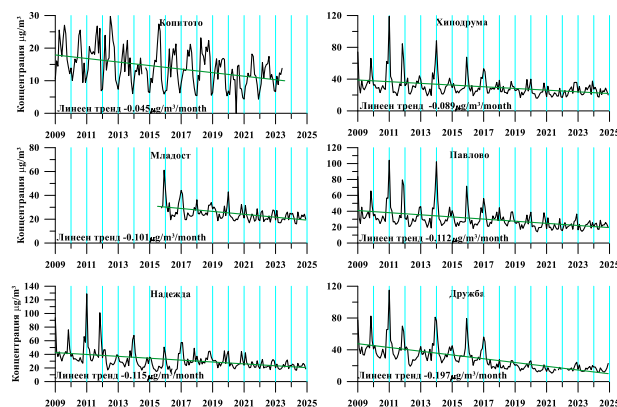
Фигура 1. Ход на средномесечните концентрации и трендове на PM 10
