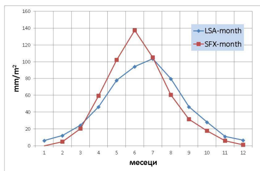
Фигура 1. Сравнение на месечното изпарение за България от SURFEX и LSA-SAF
