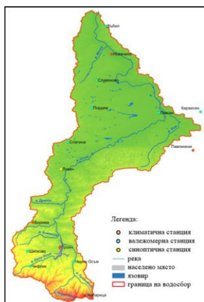
Фигура 1. Метеорологични станции във водосбора на р. Осъм
