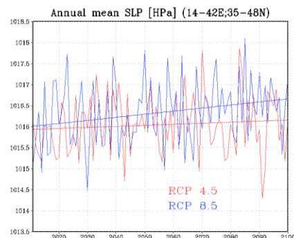
Фигура 1. Сравнение на междугодишния ход на средното налягане на морско ниво за Балканския полуостров и Черно море по моделните симулации за сценарии RCP4.5 (червено) и RCP8.5 (синьо) за периода 2011–2100 г. Дадени са и съответните линейни трендове със съответния цвят
