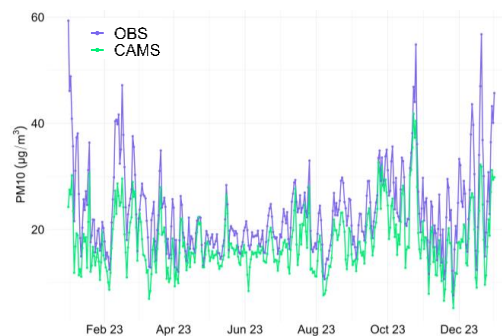
Фигура 1. Времеви ход на концентрациите на ФПЧ 10 , осреднени за 34 станции през 2023 г.
