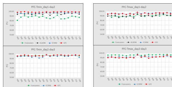
Фигура 3. PFC на прогнозите от синоптиците и от числените модели за T_{\min} и T_{\max} в отделните точки
