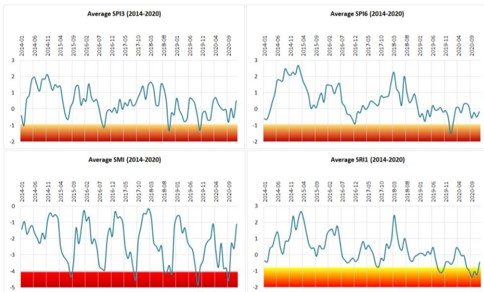
Фиг. П.2.5-12. Многогодишно изменение на средните за страната стойности на индексите, изчислени по точкови данни за периода 2014–2020 г. Степента на засушаване се определя по скала в зависимост от достигнатите прагови стойности.
