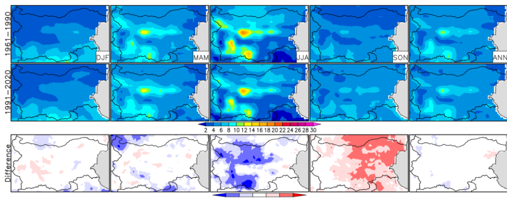
Фиг. П.2.5-4. Многогодишни средни стойности на R10mm за сезоните зима, пролет, лято и есен по данни от ERA5 Land, както и на годишна база (ANN). Абсолютните разлики на втория период спрямо първия са показани на третия ред. Единиците са брой дни.
