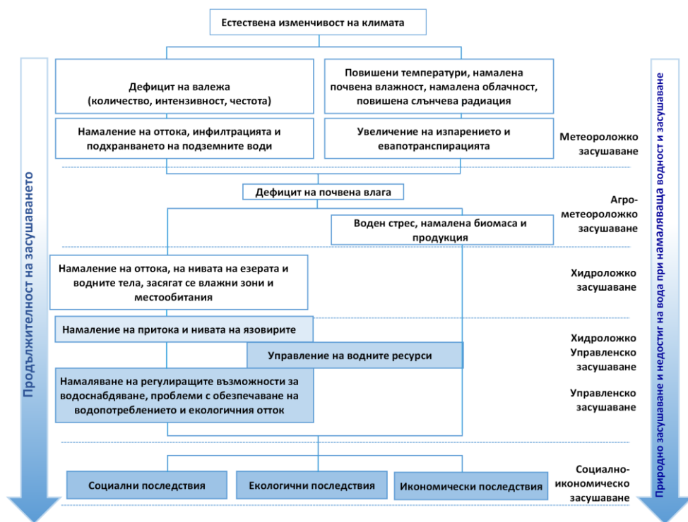
Фиг. П.2.5-11. Връзка типове – продължителност на засушаването (адаптирано по: Monzonis et al.)
